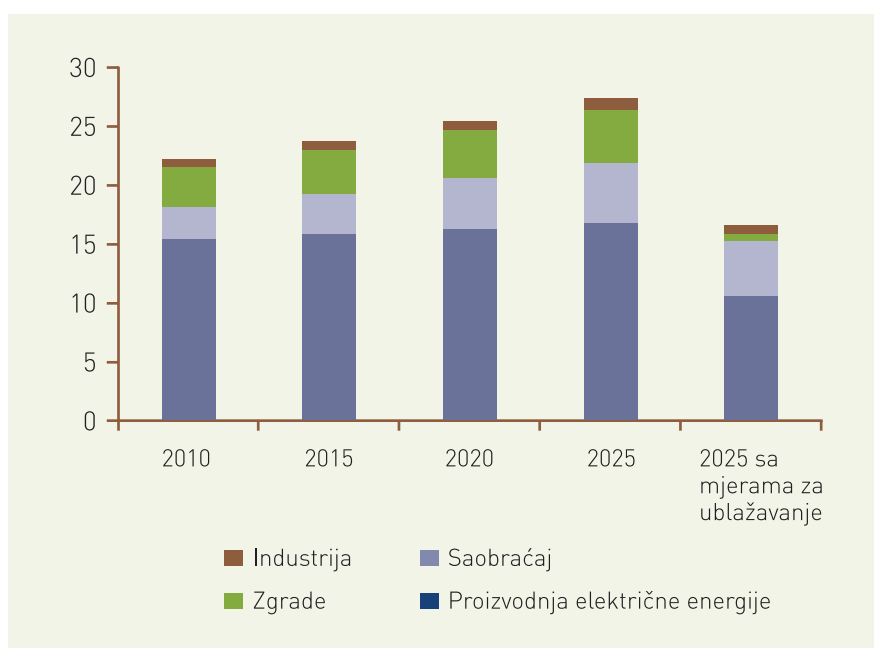
Slika 8. Približni trendovi emisija nastalih sagorijevanjem fosilnih goriva, prema sektorima, u periodu između 2010. i 2025. godine, i cjelokupni potencijal za ublažavanje klimatskih promjena u 2025. godini
